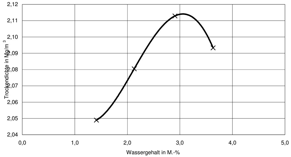
Proctorkurve des Baustoffgemisches 0/45 (STS) gemäß Prüfzeugnis Nr. 44725SoB/23 vom 19.01.2024
