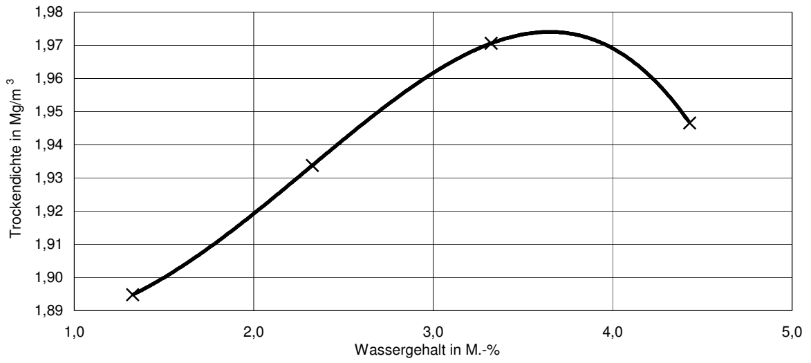
Proctorkurve des Baustoffgemisches 0/32 (STS) gemäß Prüfzeugnis Nr. 44723SoB/23 vom 19.01.2024
