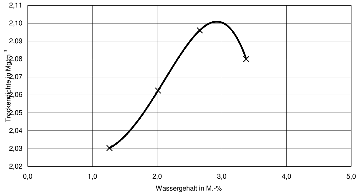
Proctorkurve des Baustoffgemisches 0/45 (FSS - UF 3) gemäß Prüfzeugnis Nr. 44727SoB/23 vom 19.01.2024
