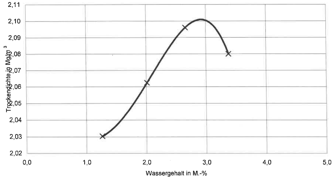
Proctorkurve des Baustoffgemisches 0/45 (FSS - UF 3)
